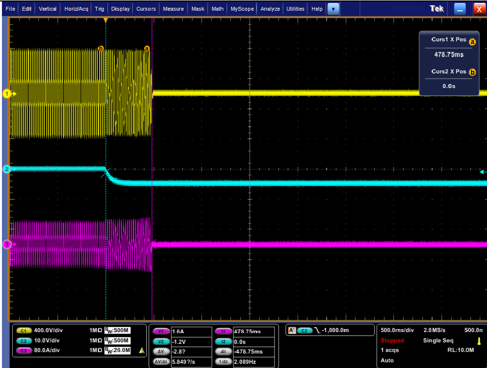
PEUT 100, PAC -10, QAC 5, = 478.75ms
